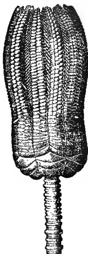
ENCRINURUS MONILIFORMIS. (Trias.)
